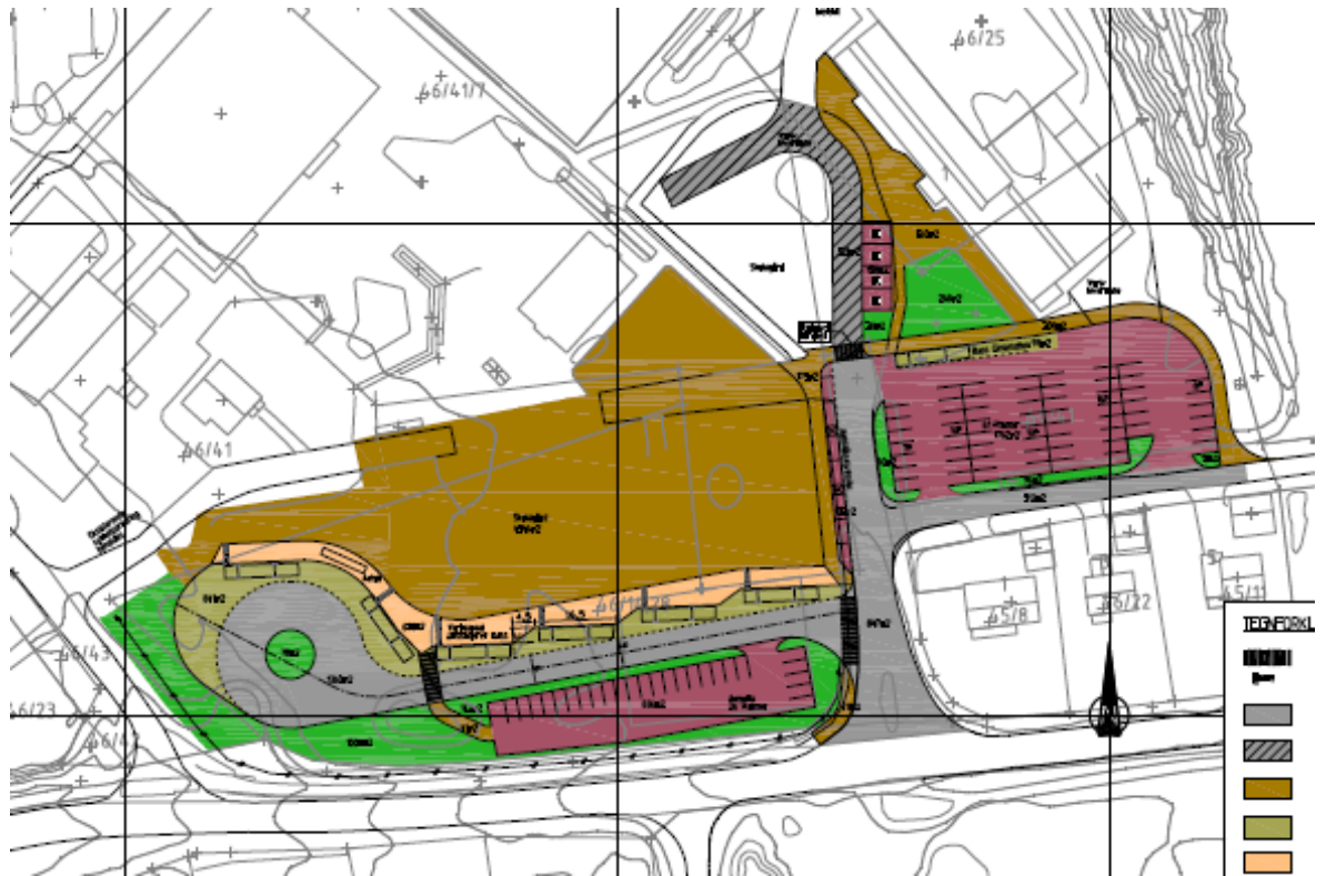
Oversiktstegning tidligere skisse trafikkløsning
